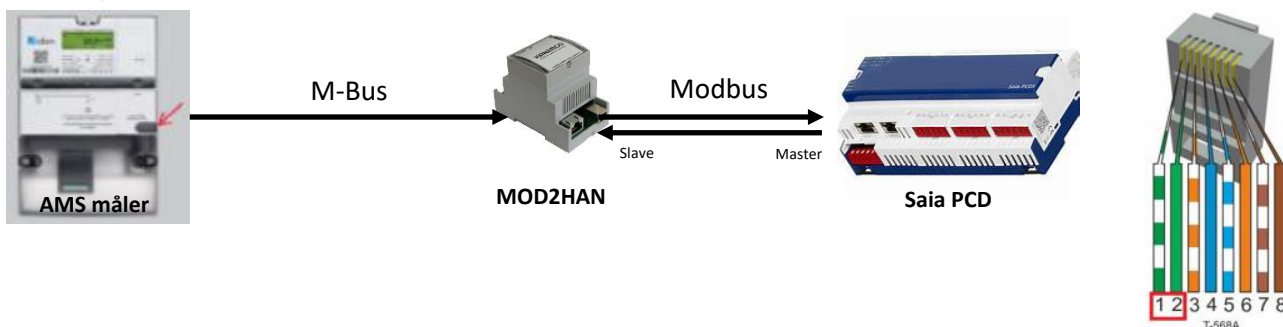
Fig. RJ45 – Pin1 og Pin2 for MBUS
